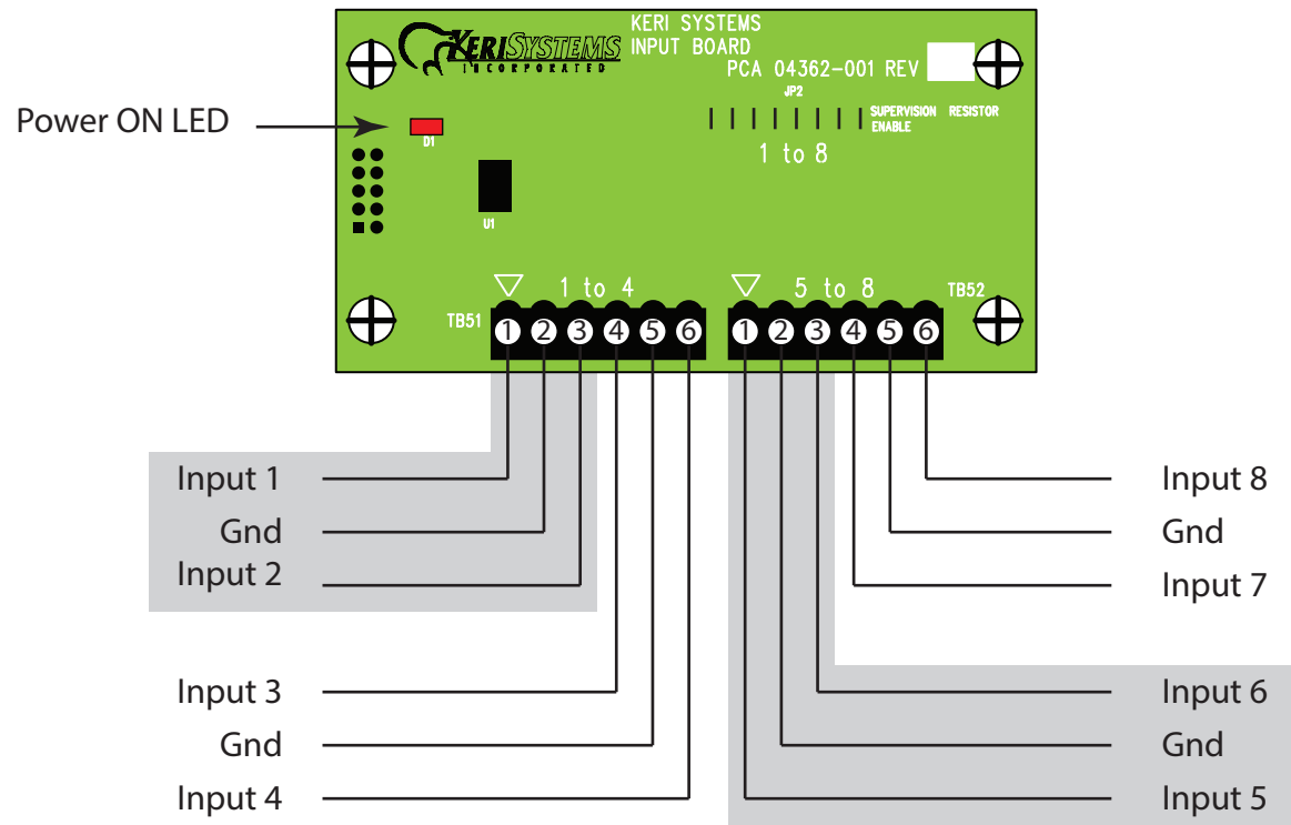
01270-004 Rev. A GIOX Input Board Wiring
