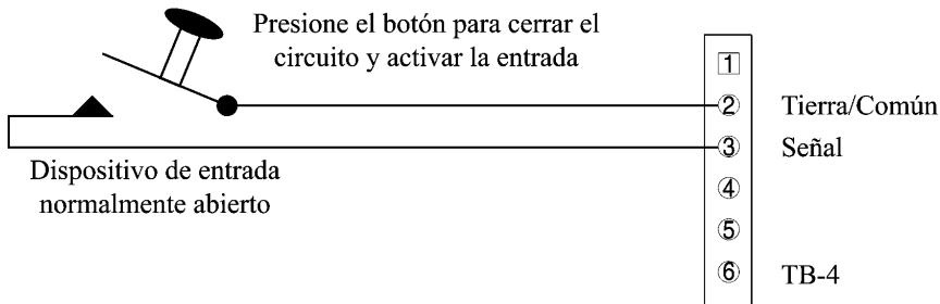
Figura 8: Conexión del pulsador de petición de salida (RTE)
