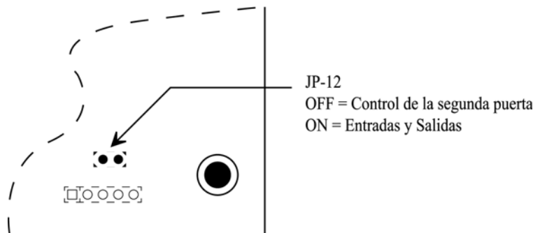
Figura 1: Puente JP12
